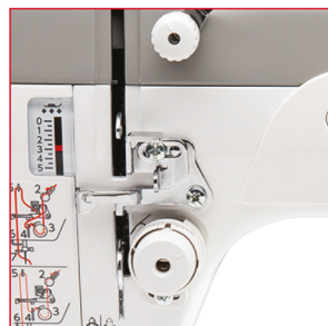
Guía de hilos pesados (HWTG)
