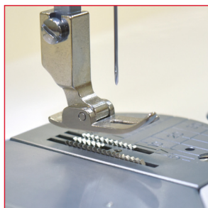
Diente de arrastre y placa de agujas tipo industrial
